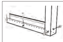
9 DETALLE DEL CANAL BASE Tres sujetadores por marco doble típico - 24" O.C. para paredes fijas
