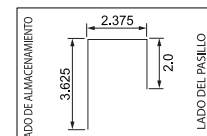
14 CANAL DEL SOMBRERO DE COPA
