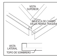
10 DETALLE DE LA ESQUINA DEL SOMBRERO DE ALTA Adjunte el ángulo interno con tornillos TEK de #10 x 3/4" en la intersección de los canales superiores.
