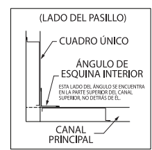
11 DETALLE DE ESQUINA INTERNA Fije el ángulo interior con tornillos TEK de #10 x 3/4" de arriba hacia abajo en incrementos de 2.0', 4.0' y 6.0'. Fije el ángulo inicial con tornillos TEK de #10 x 3/4" de arriba hacia abajo en incrementos de 2.0', 4.0' y 6.0'.
