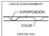
8 M-PANEL DETALLE DE SOLAPAMIENTO
